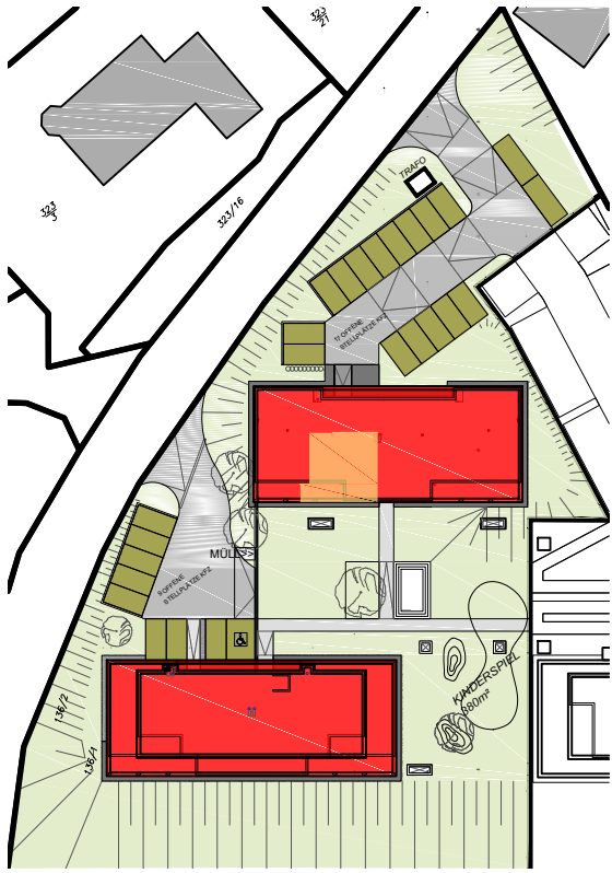
LAGEPLAN M 1:1000
