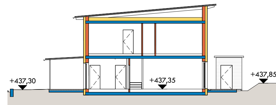
Schnitt H 3
