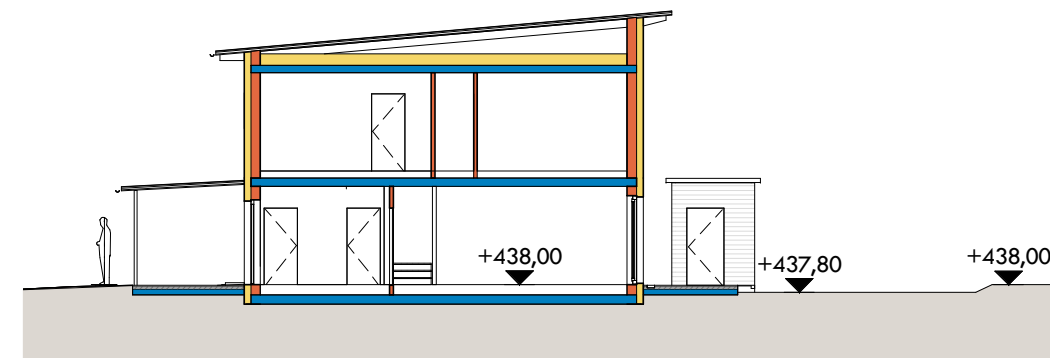
Schnitt H 10
