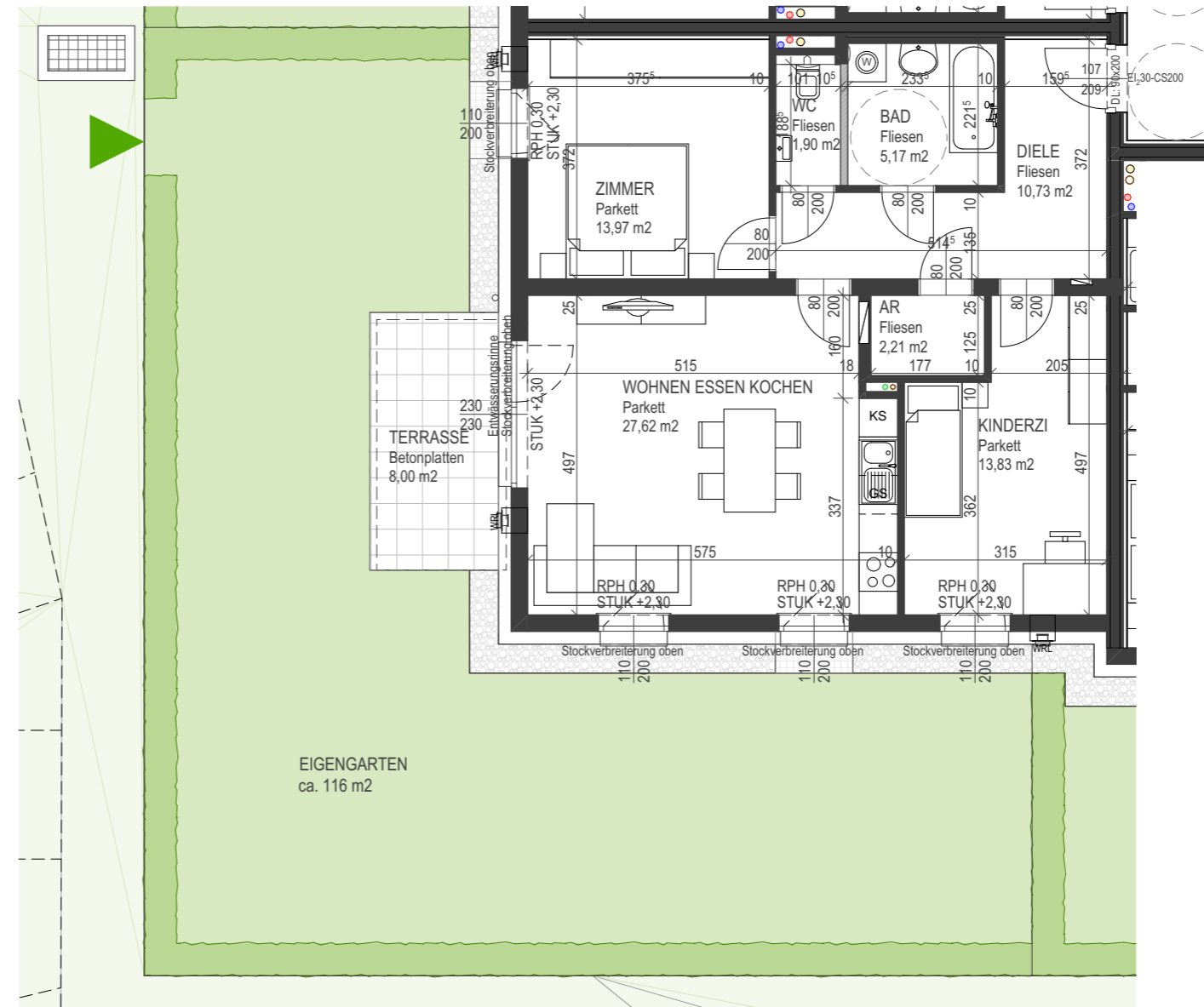
Grundriss Erdgeschoß 1:100
