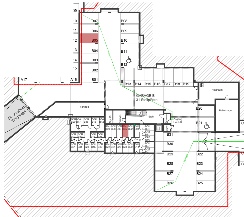
Tiefgaragenübersicht 1:500
