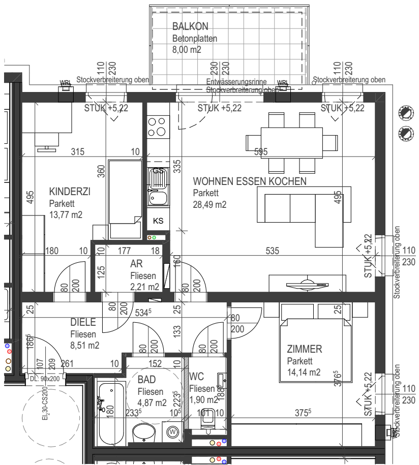
Grundriss 1. Obergeschoß 1:100
