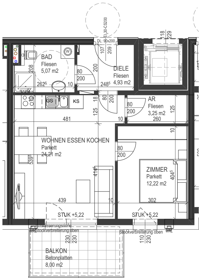
Grundriss 1. Obergeschoß 1:100
