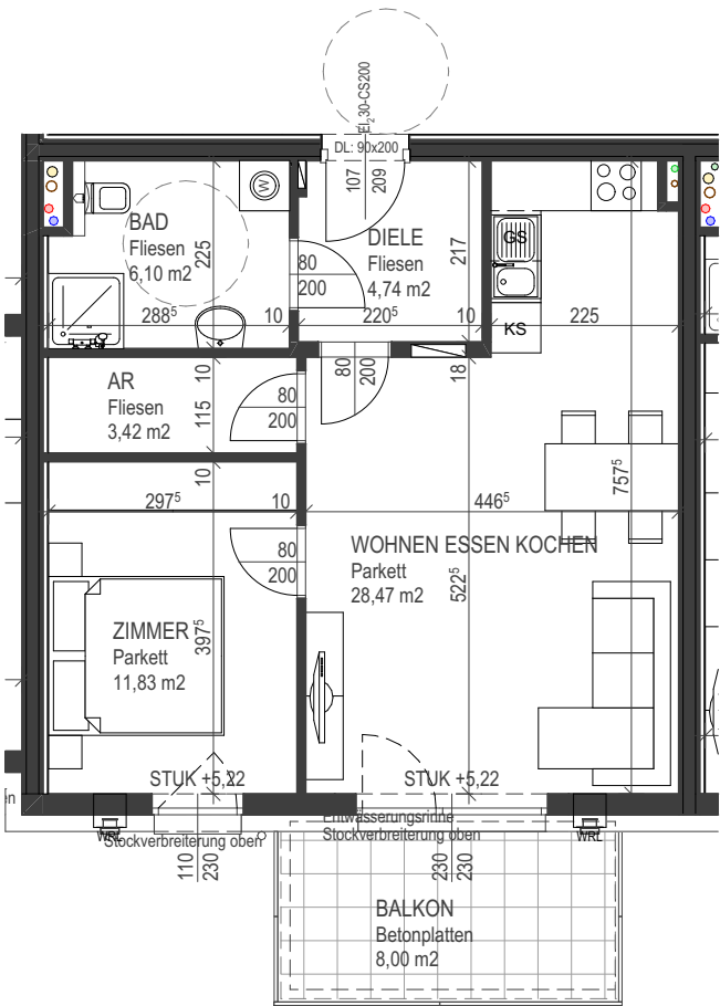
Grundriss 1. Obergeschoß 1:100
