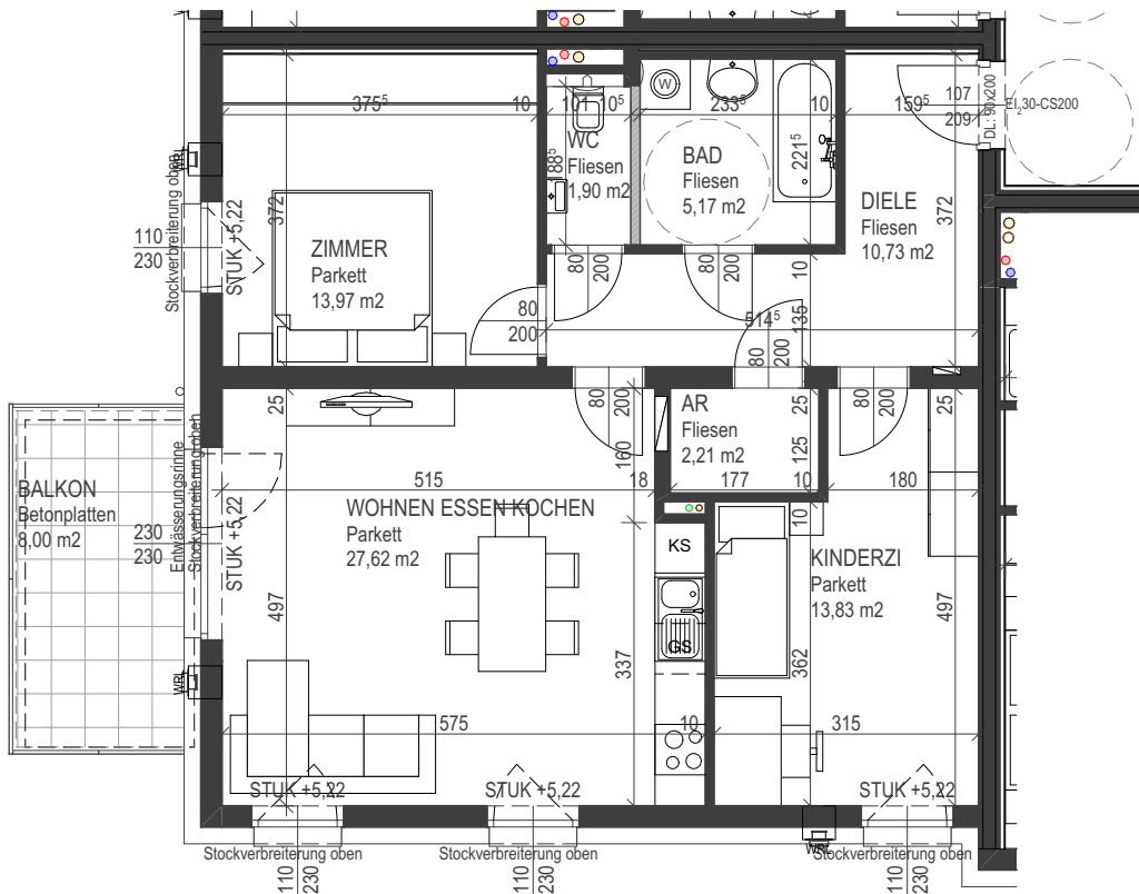
Grundriss 1. Obergeschoß 1:100
