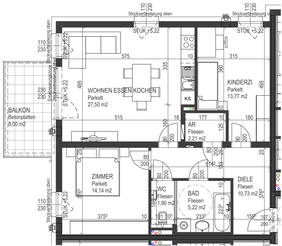
Grundriss 1. Obergeschoß 1:100
