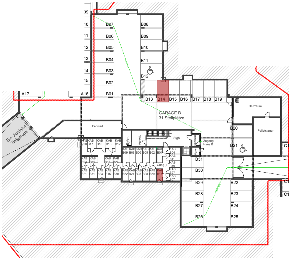
Tiefgaragenübersicht 1:500
