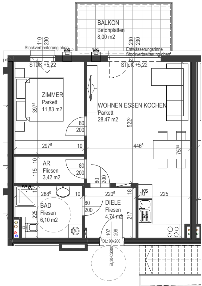
Grundriss 1. Obergeschoß 1:100
