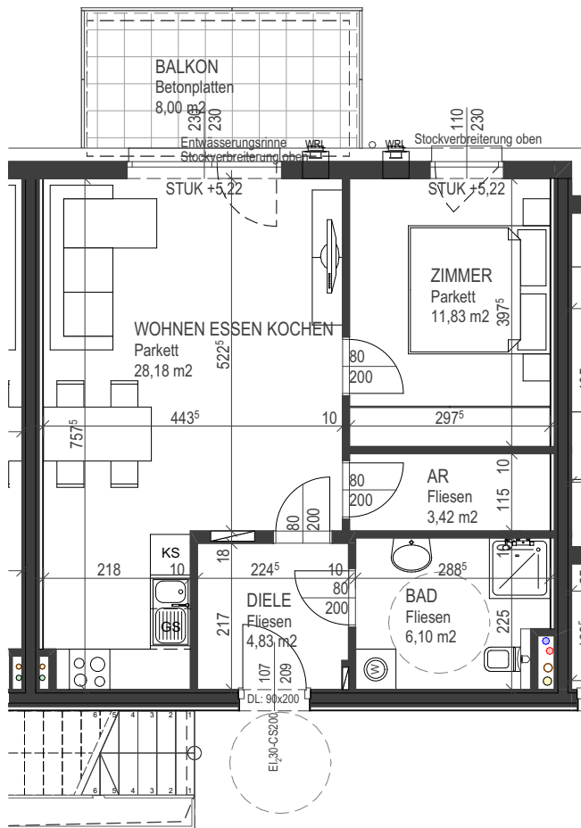
Grundriss 1. Obergeschoß 1:100
