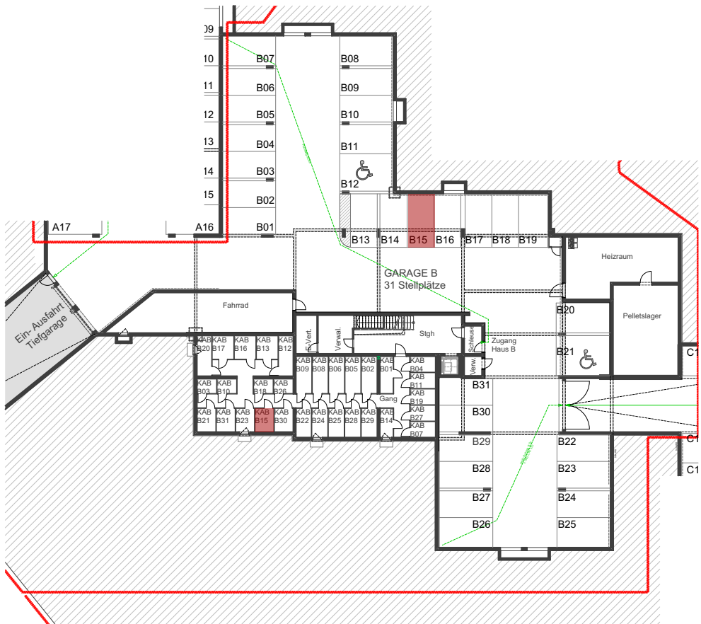
Tiefgaragenübersicht 1:500
