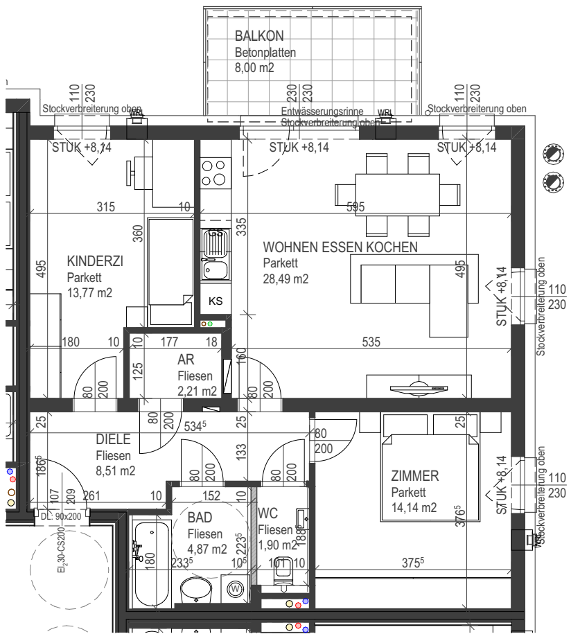
Grundriss 2. Obergeschoß 1:100
