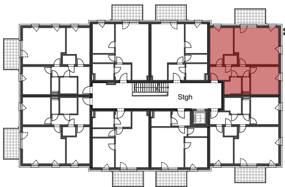
Geschoßübersicht 2.OG 1:500
