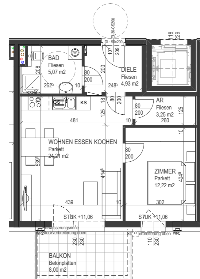
Grundriss 3. Obergeschoß 1:100
