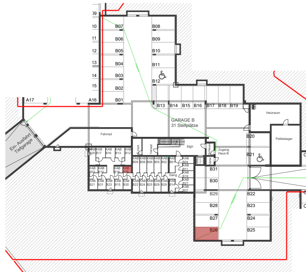
Tiefgaragenübersicht 1:500
