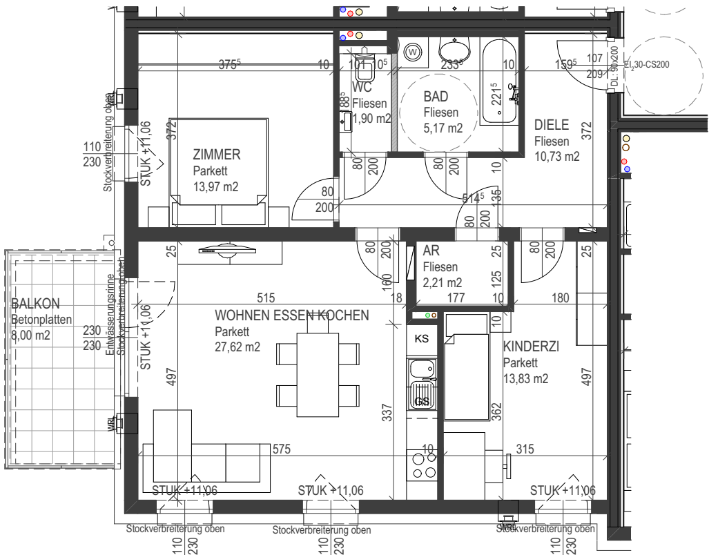
Grundriss 3. Obergeschoß 1:100
