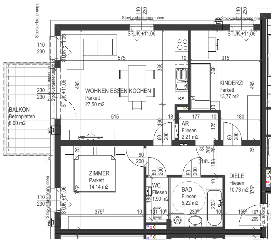
Grundriss 3. Obergeschoß 1:100
