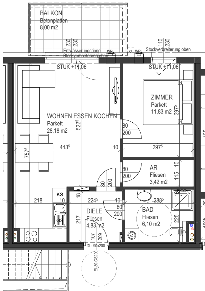
Grundriss 3. Obergeschoß 1:100
