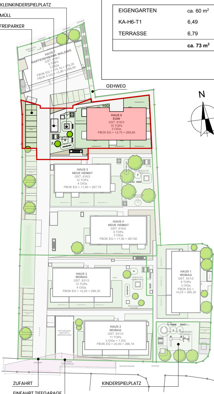
ÜBERSICHTSPLAN 1:1000
