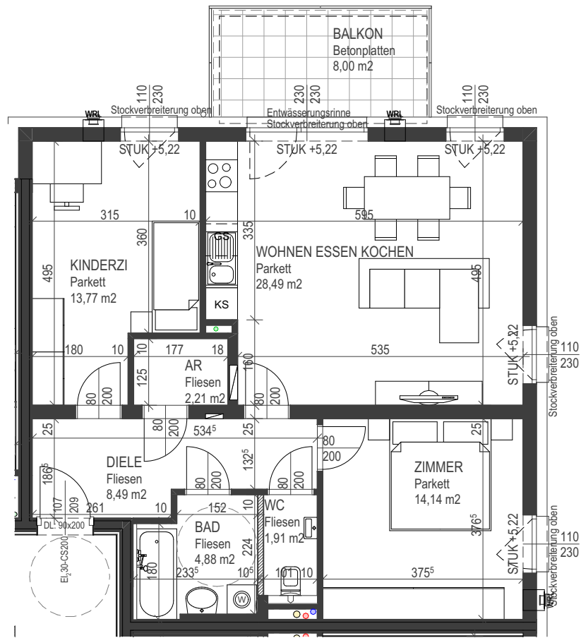
Grundriss 1. Obergeschoß 1:100
