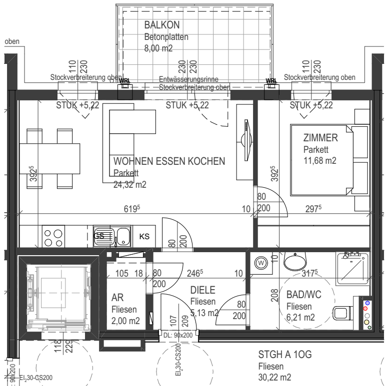
Grundriss 1. Obergeschoß 1:100
