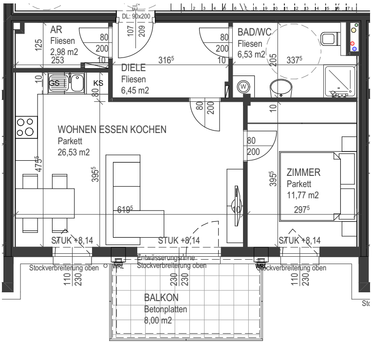
Grundriss 2. Obergeschoß 1:100
