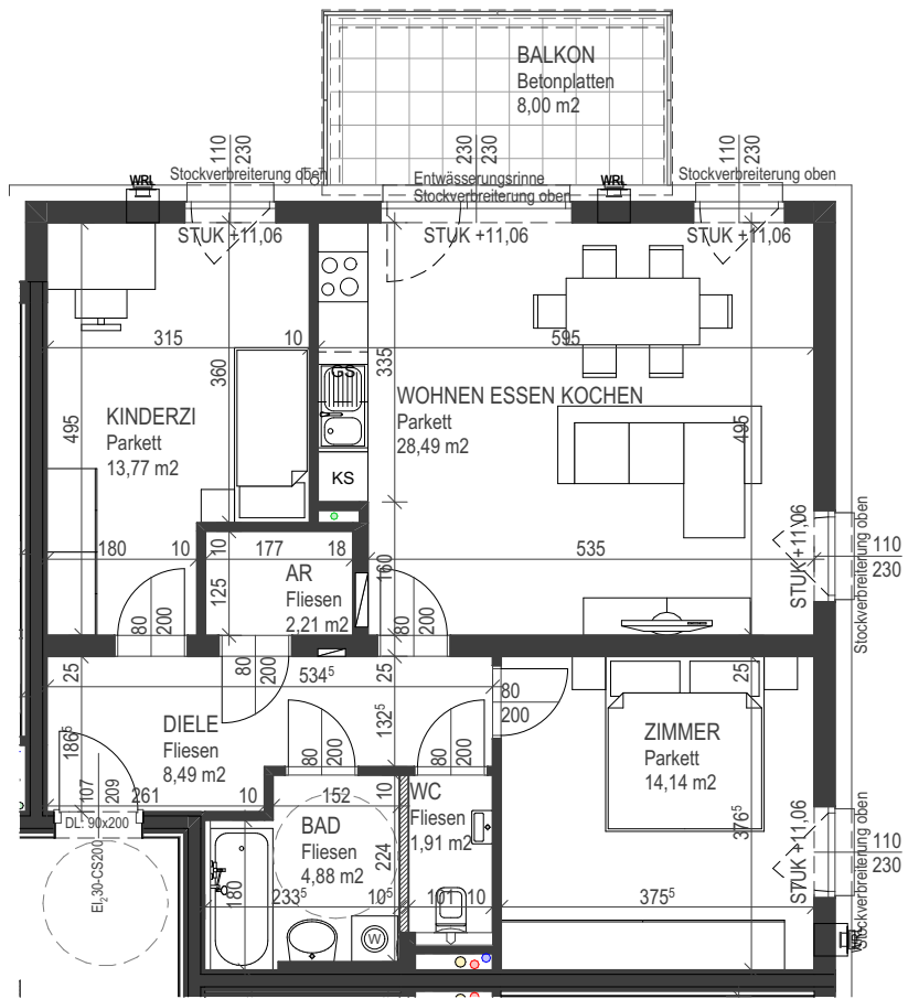
Grundriss 3. Obergeschoß 1:100
