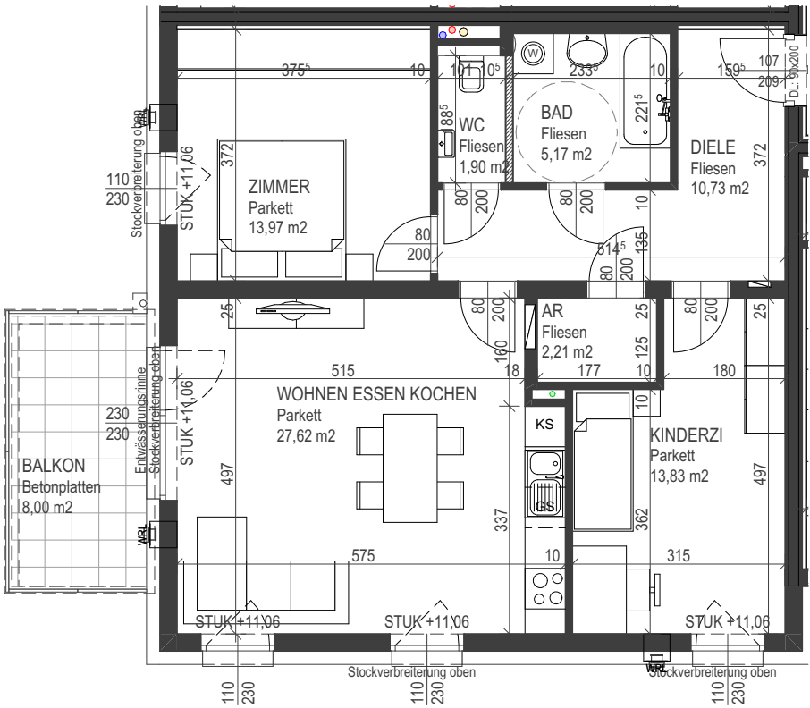
Grundriss 3. Obergeschoß 1:100
