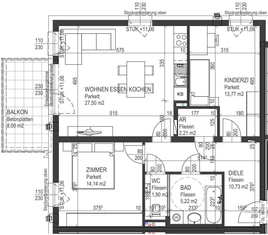
Grundriss 3. Obergeschoß 1:100
