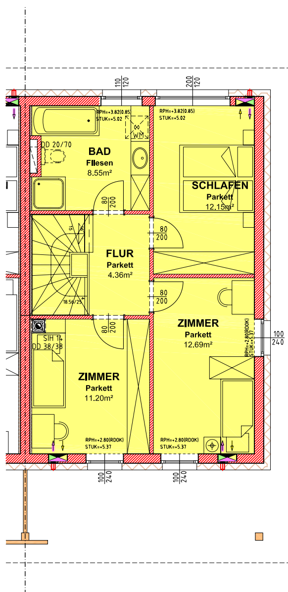
OBERGESCHOSS
