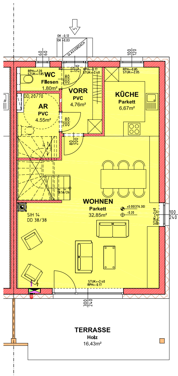
ERDGESCHOSS
