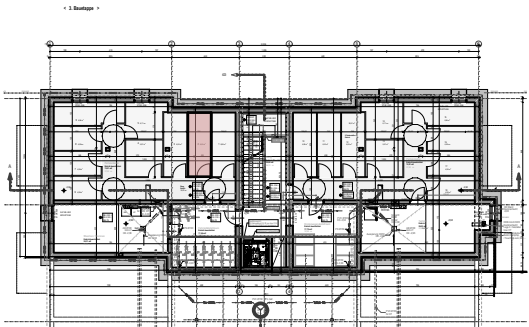
ÜBERSICHT KELLERGESCHOSS
