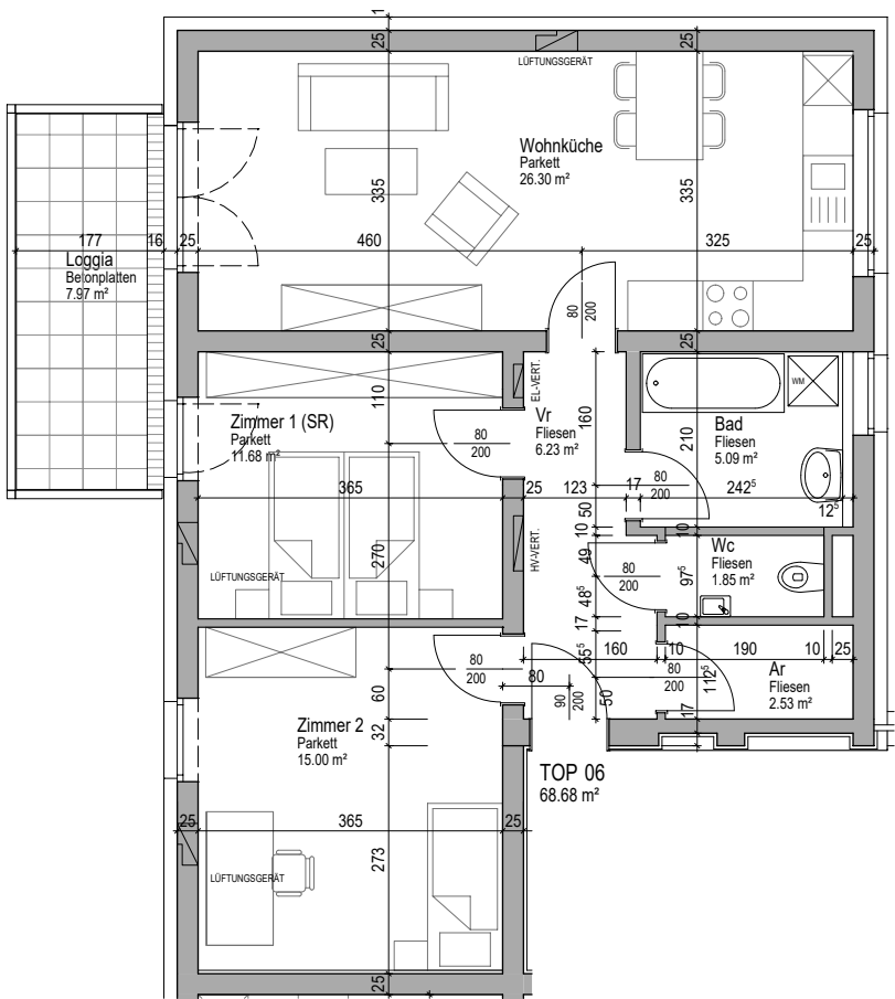
Grundriss 1 : 100
