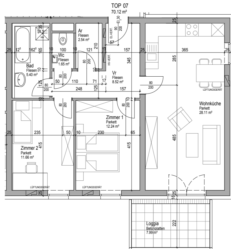
Grundriss 1 : 100
