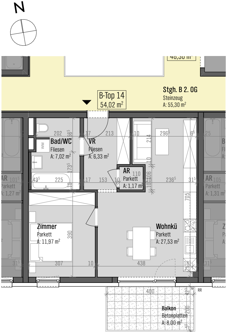
2. OBERGESCHOSS | M 1:100
