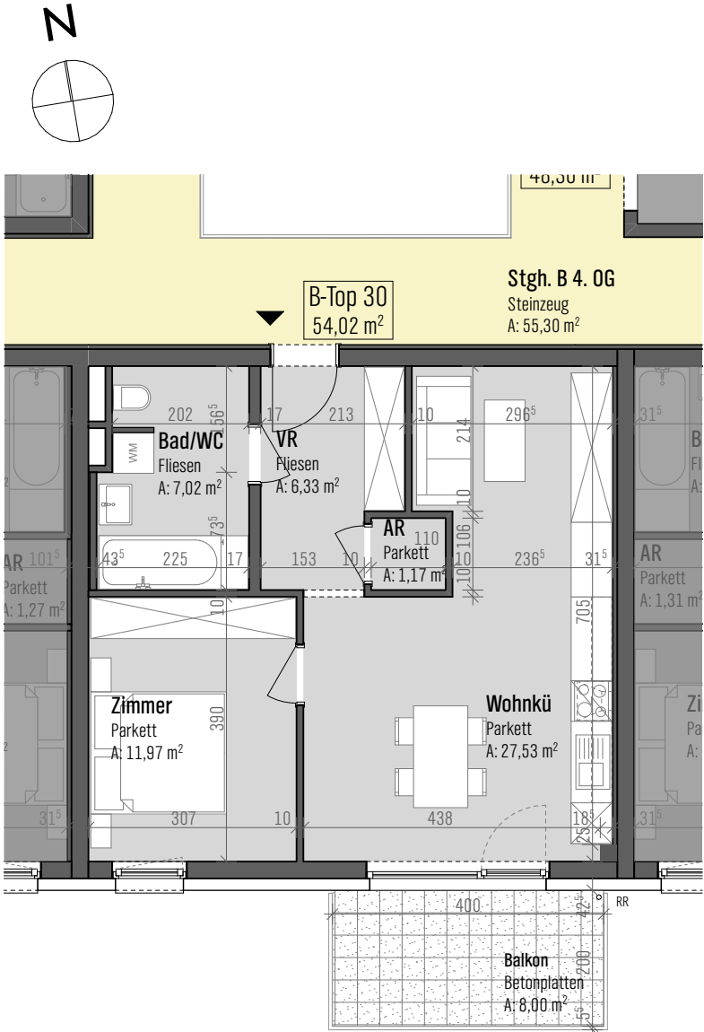
4. OBERGESCHOSS | M 1:100
