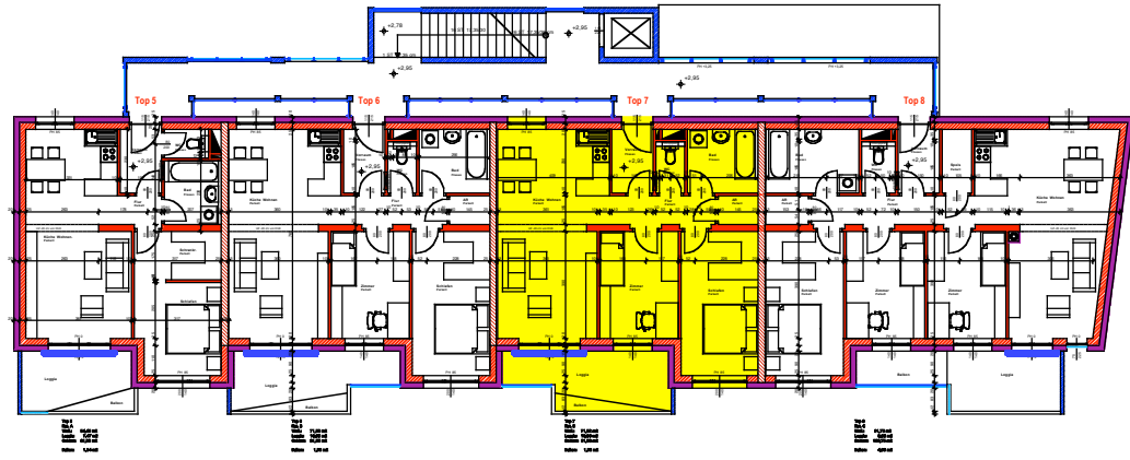
1. Obergeschoß
