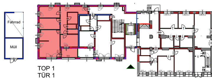
Erdgeschoss Übersicht - Wohnung
