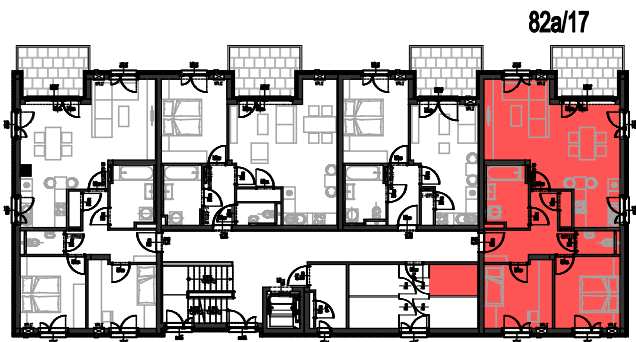
1.OBERGESCHOSS ÜBERSICHT
