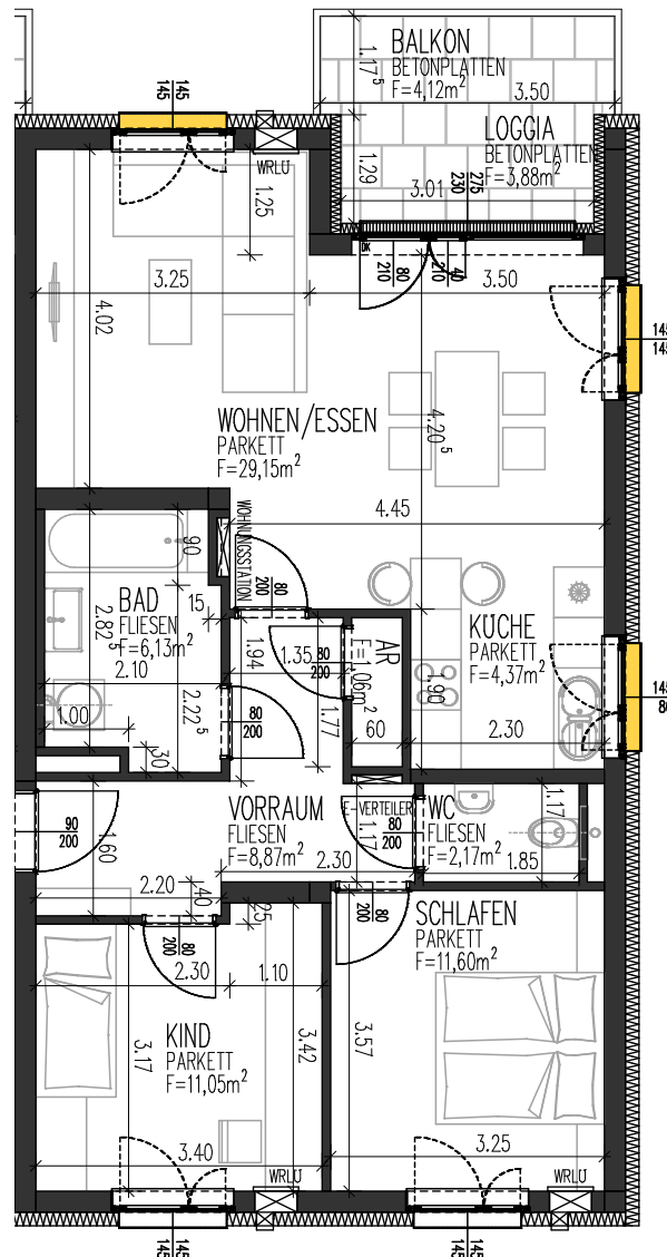
1.OBERGESCHOSS 82a/17
