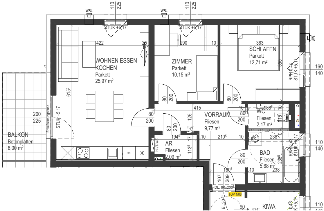
Grundriss 1.Obergeschoß 1:100
