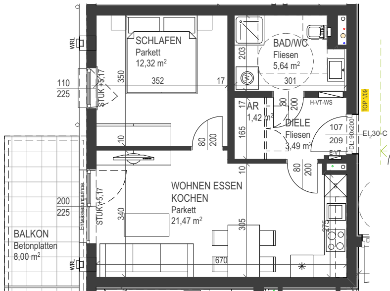
Grundriss 1.Obergeschoß 1:100
