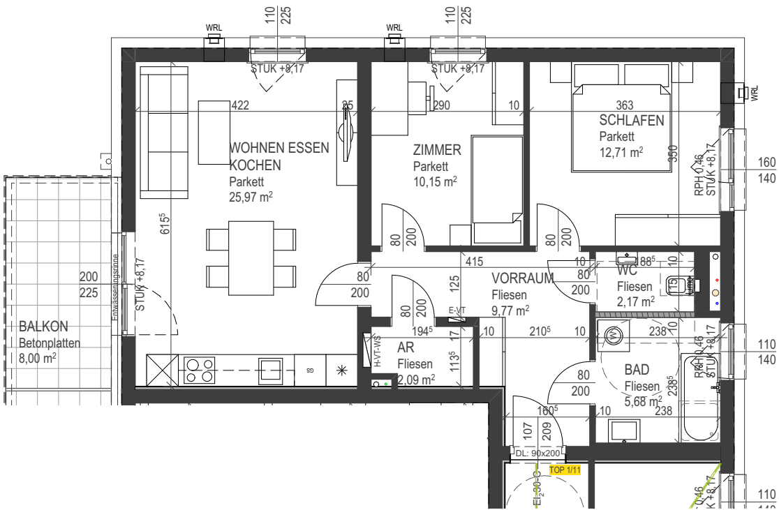
Grundriss 2.Obergeschoß 1:100
