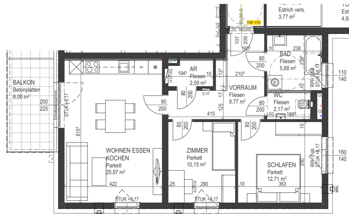
Grundriss 2.Obergeschoß 1:100
