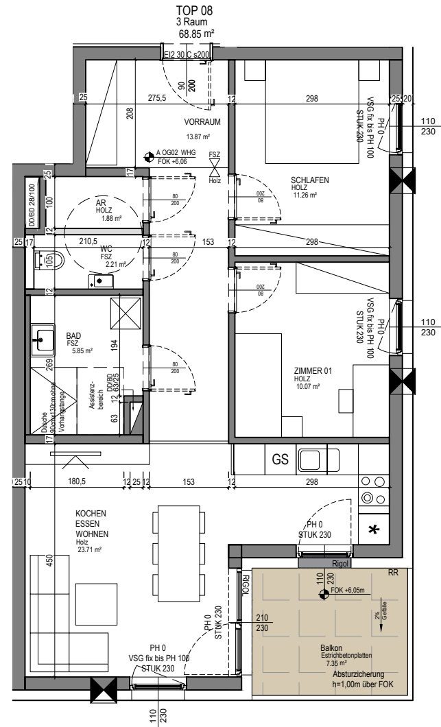
WOHNUNGSGRUNDRISS M 1:100
