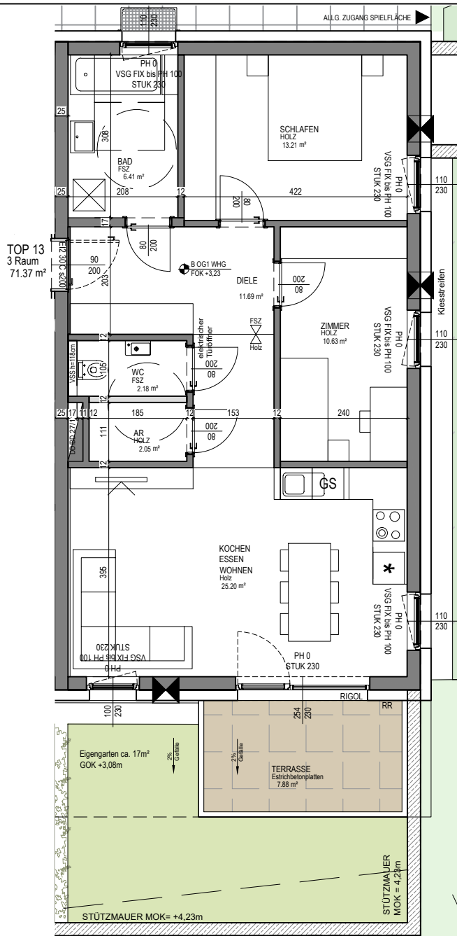
WOHNUNGSGRUNDRISS M 1:100
