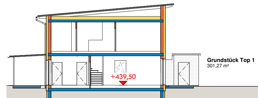
SCHNITT M 1 : 200
