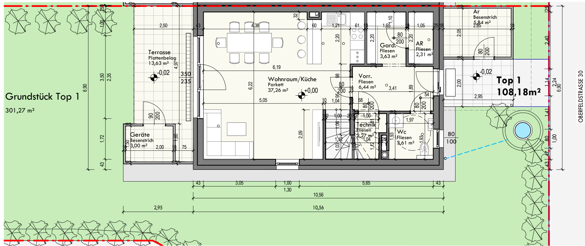
EG M 1 : 100
