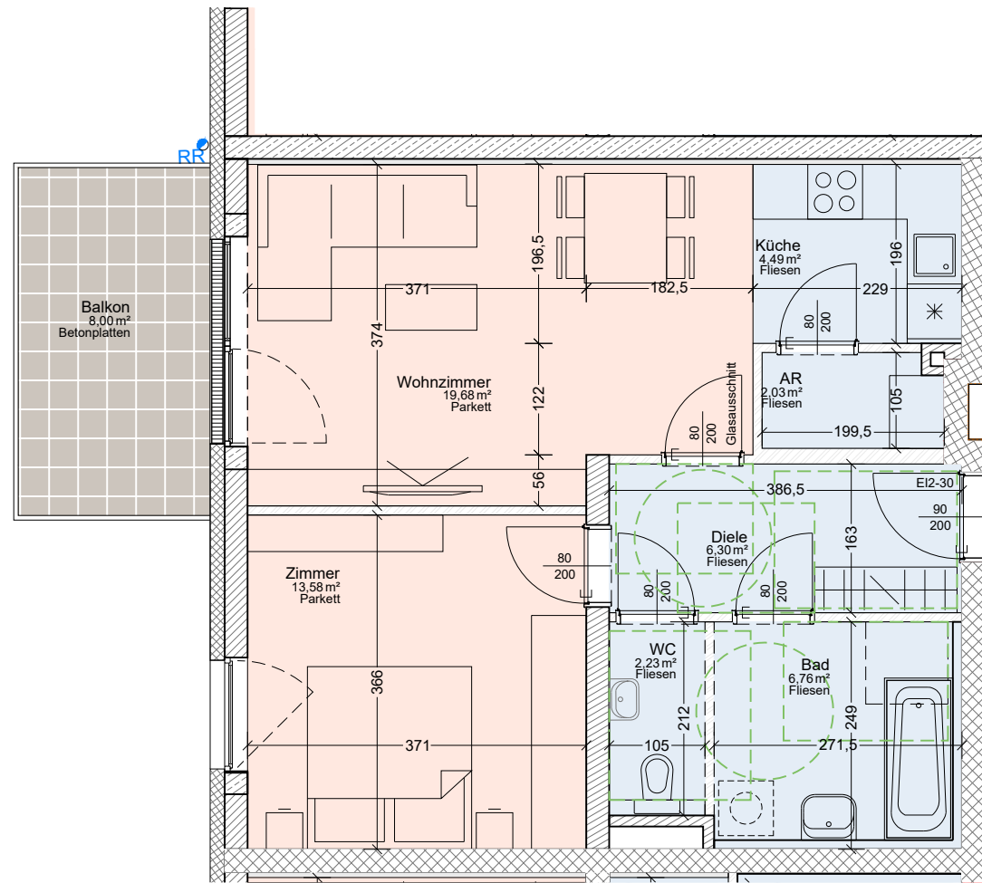
2.OBERGESCHOSS TOP 10 - A.10
