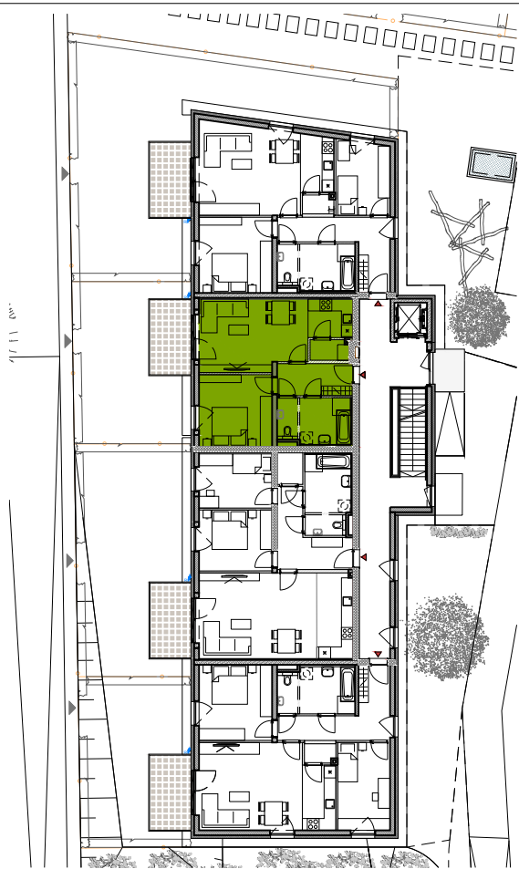
GESCHOßÜBERSICHT 2.OBERGESCHOSS HAUS A
