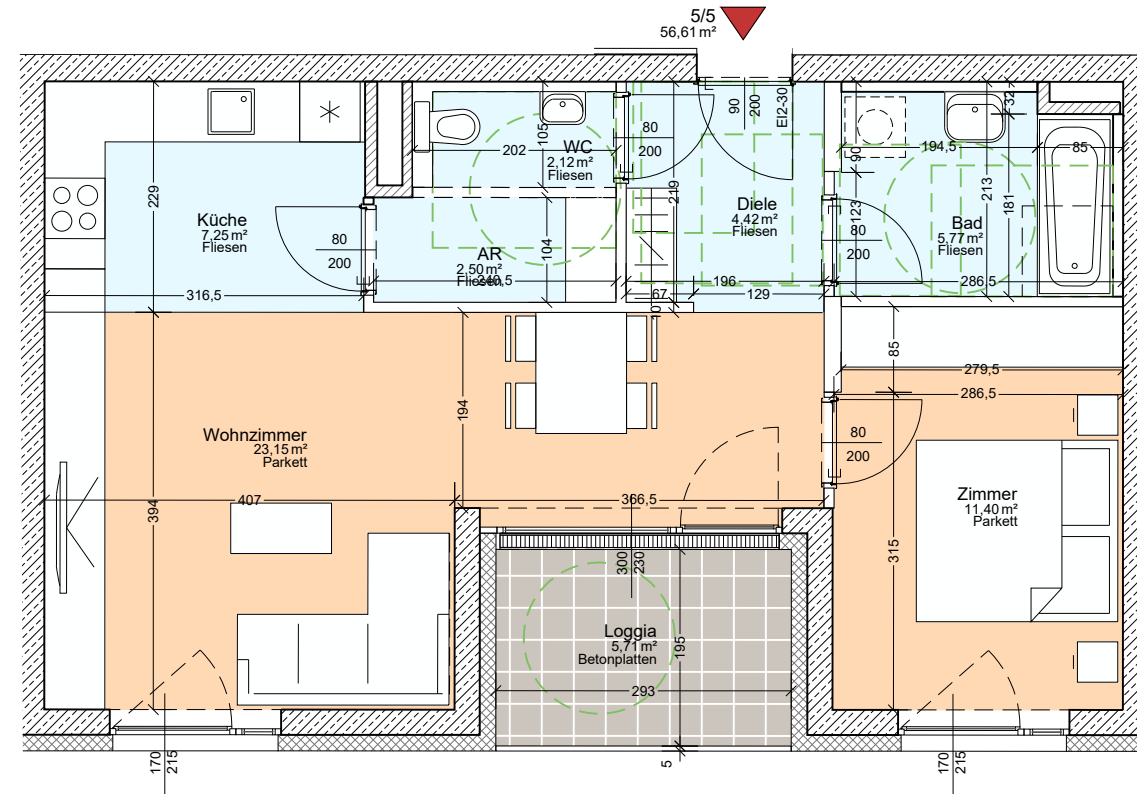
1.OBERGESCHOSS Haus D1/Top5/ Tür 5 M 1:75 @ DIN A3
