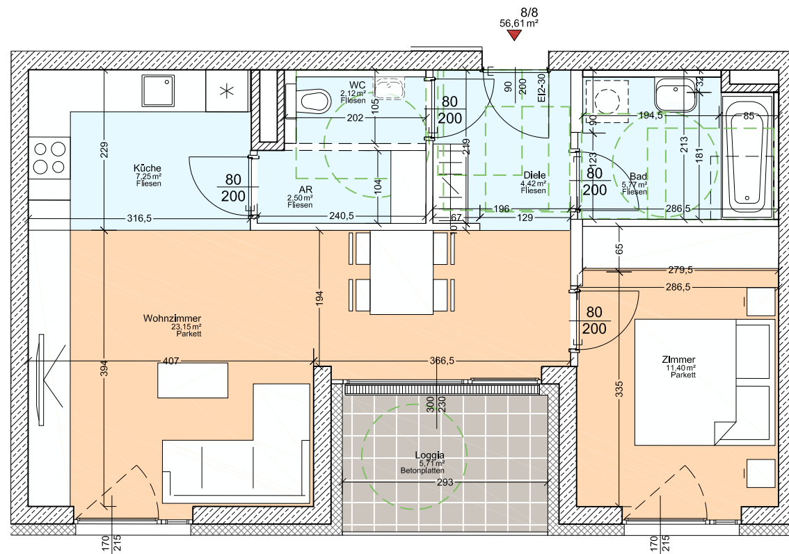
2.OBERGESCHOSS Haus D1/Top 8/ Tür 8 M 1:75 @ DIN A3
