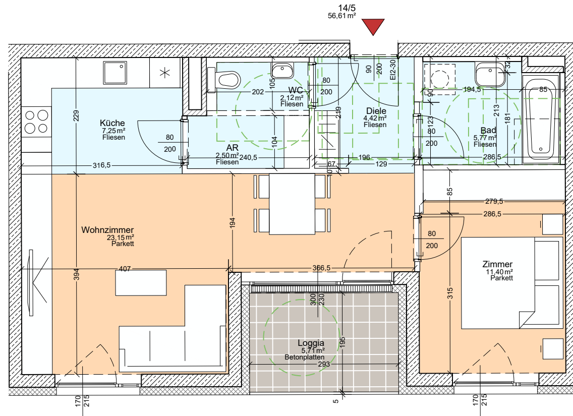
1.OBERGESCHOSS Haus D2/Top14/Tür 5 M 1:75 @ DIN A3
