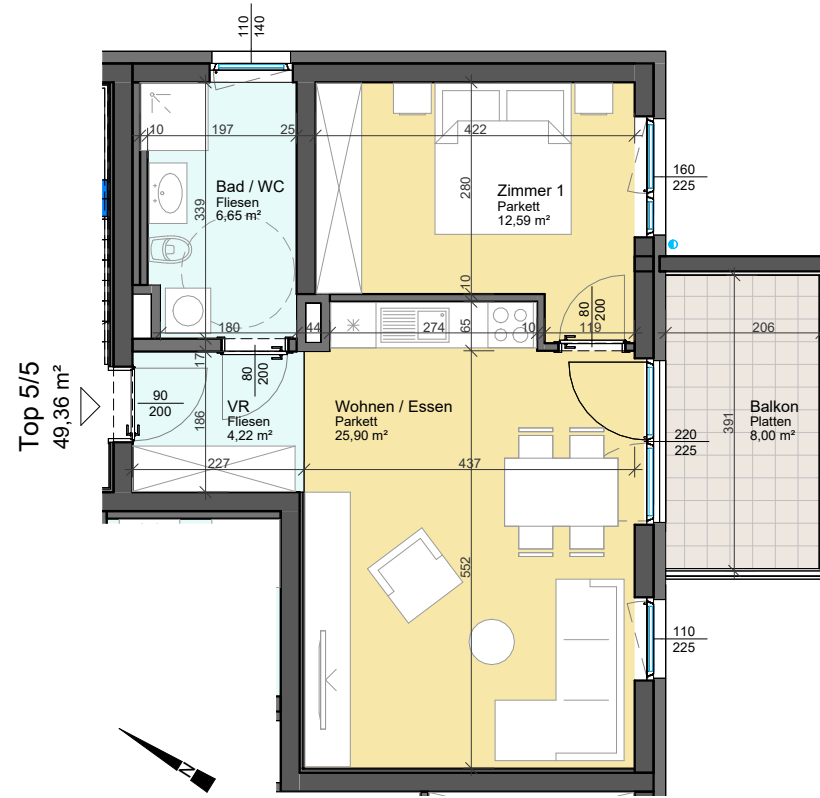
1. OBERGESCHOSS Am Nordsaum 82d - Haus 5 - Top 5/5
