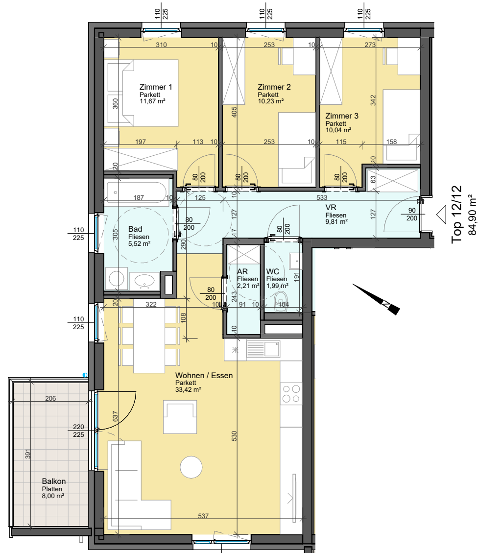
2. OBERGESCHOSS Am Nordsaum 82d - Haus 5 - Top 12/12
