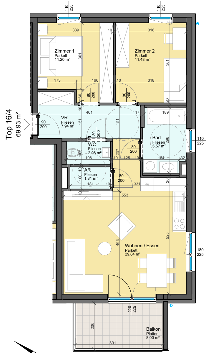
1. OBERGESCHOSS Am Nordsaum 82c - Haus 6 - Top 16/4
