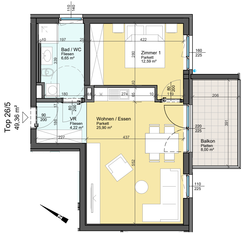
1. OBERGESCHOSS Am Nordsaum 82b - Haus 7 - Top 26/5
