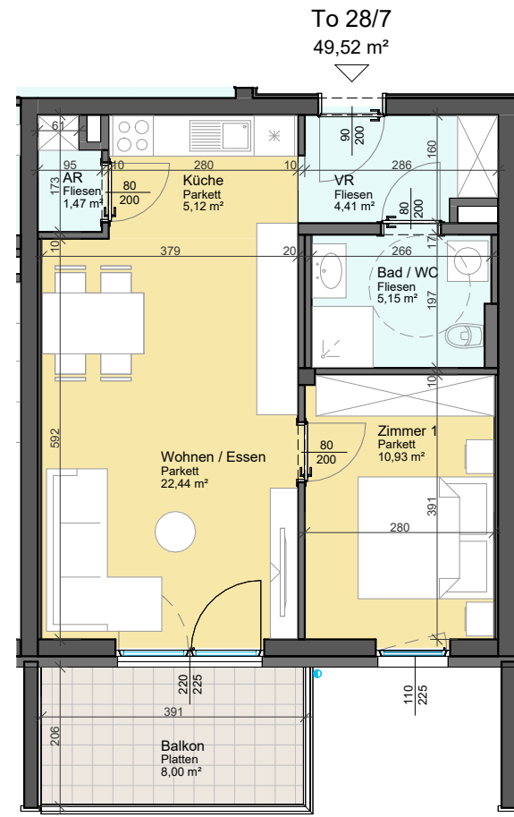
1. OBERGESCHOSS Am Nordsaum 82b - Haus 7 - Top 28/7
