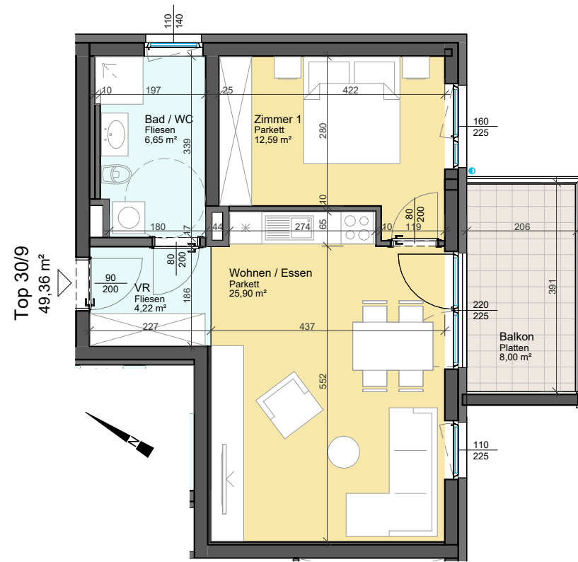
2. OBERGESCHOSS Am Nordsaum 82b - Haus 7 - Top 30/9
