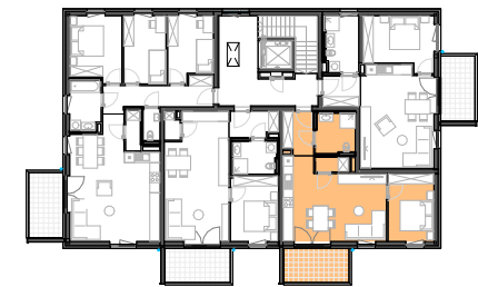
ÜBERSICHT GESCHOSS
